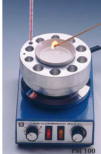
PM-Thermoblock auf Magnetrührer
